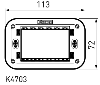
4 MODÜL KAİDE
