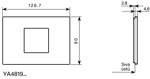
3 modül ortalanmış çerçeve
