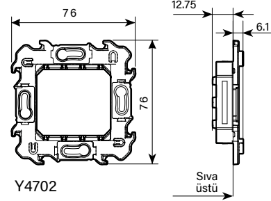
2 modül kaide
