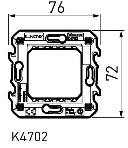
3 MODÜL KAİDE
