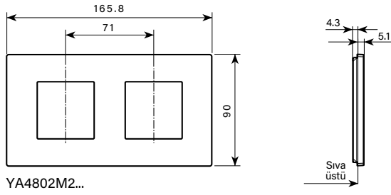
2+2 modül çerçeve, 71 mm merkez aralığı – yatay/dikey kullanım
