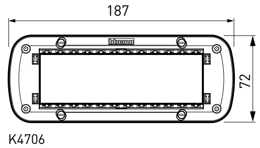
6 MODÜL KAİDE
