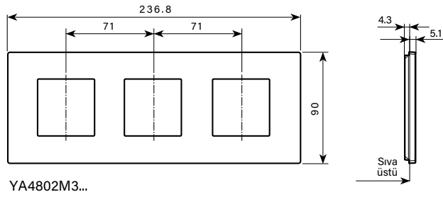
2+2+2 modül çerçeve, 71 mm merkez aralığı – yatay/dikey kullanım
