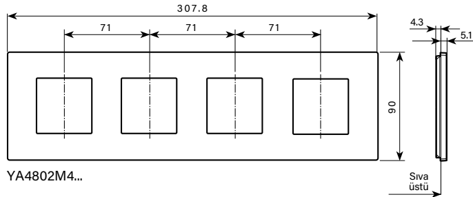
2+2+2+2 modül çerçeve, 71 mm merkez aralığı – yatay/dikey kullanım
