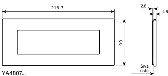
7 modül çerçeve
