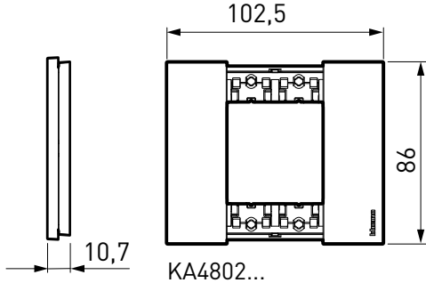
2 MODÜL ÇERÇEVE
