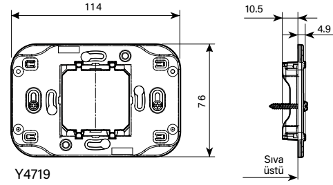
2 modül ortalanmış kaide
