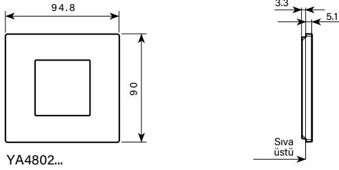
2 modül çerçeve
