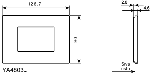
3 modül çerçeve
