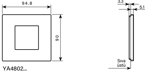
2 modül çerçeve
