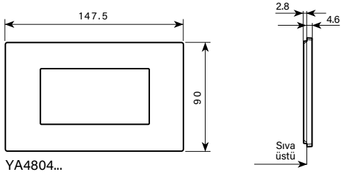
7 modül çerçeve
