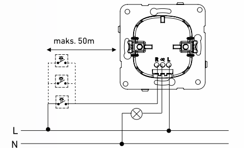
Light Anahtarlı Çoklu Kullanımı
